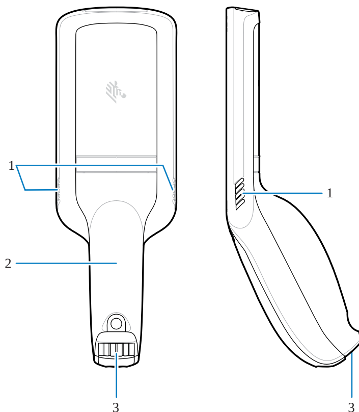
Figura 2 Vista laterale e posteriore
