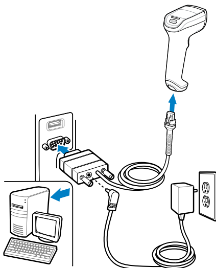
Connessione RS-232 DS8208/R cablato
