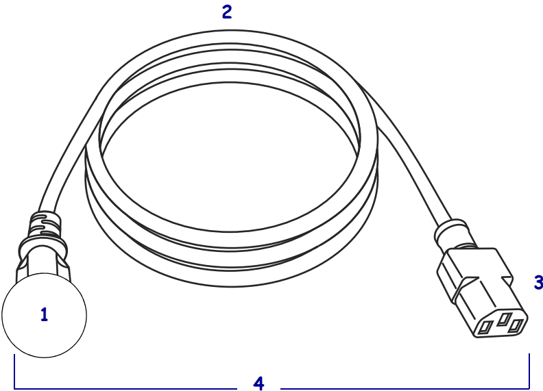
Figura 9 • Specifiche del cavo di alimentazione
