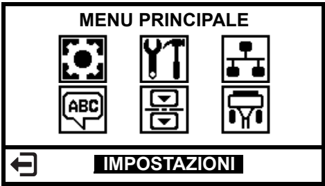
Figura 6 • Menu principale
