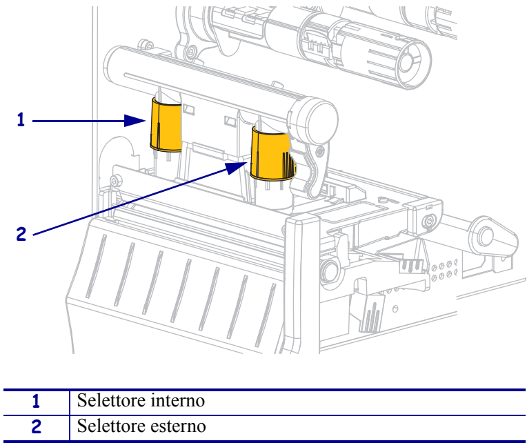
Figura 11 • Selettori di regolazione della pressione della testina di stampa
